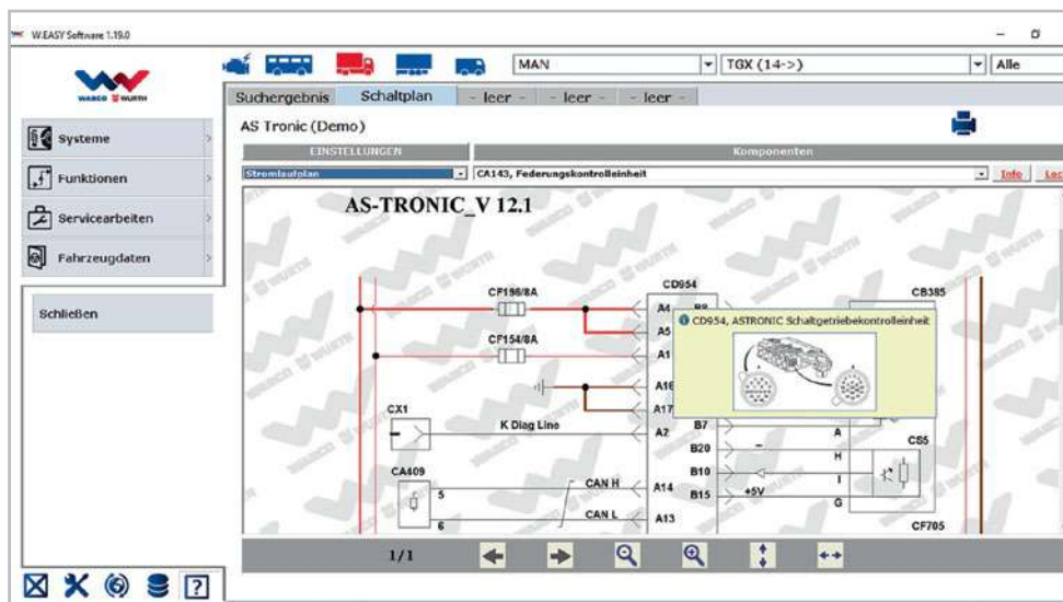
Interaktive eldiagrammer
